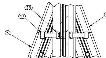
G ( 1 : 2 ) Detail spojení šikmé vzpěry
