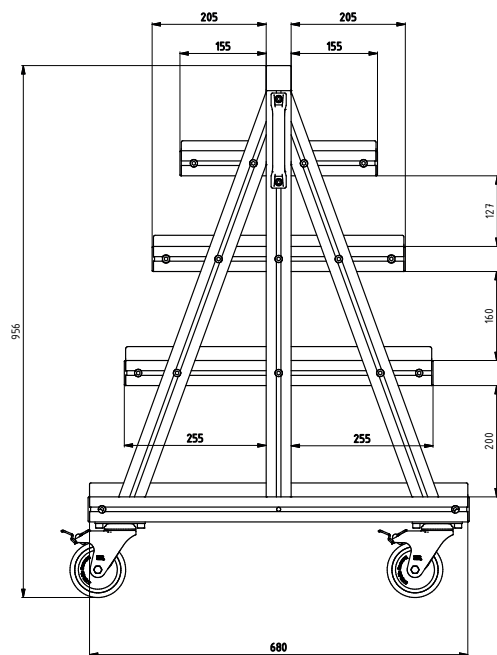
E-E ( 1 : 6 )
