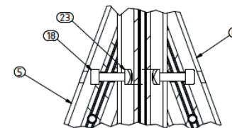
G (1:2) Detail spojení šikmé vzpěry
